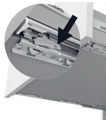
Smontaggio facilitato: premere le linguette sotto il cassetto e sfilarlo dalle guide Easy disassembly: press the tabs underneath the drawer and slide it off the rails.
