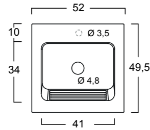
Cod. 855
