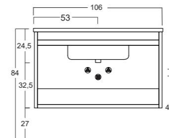
COD.232106
