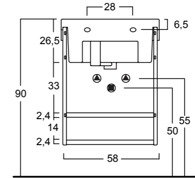
Cod. 21ML60 - 965
