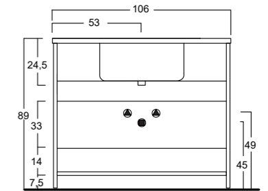
COD.23Z106
