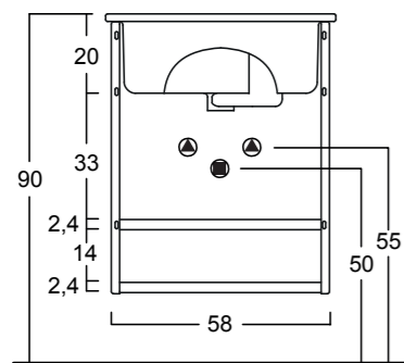
Cod. 21ML60 - 865
